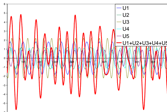
Abbildung 12: Rauschähnliches Signal mit Crestfaktor 11 dB
